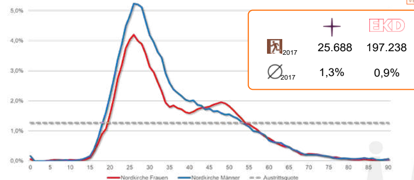
Abbildung 5: Austrittswahrscheinlichkeit 2017
